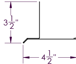
SOFFIT TRIM
